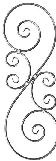
29503 Ø12 mm 310x900 mm 4,01 kg
