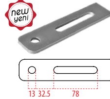
Denge Sacı Guide Plate
