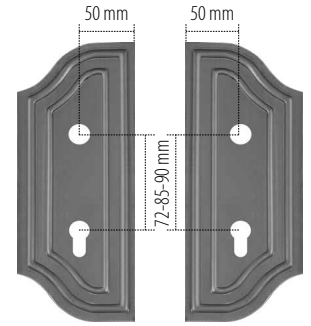
3951-A 105x265 mm 2 mm
