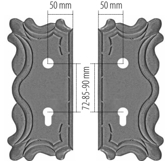
3957-A 135x305 mm 3 mm
