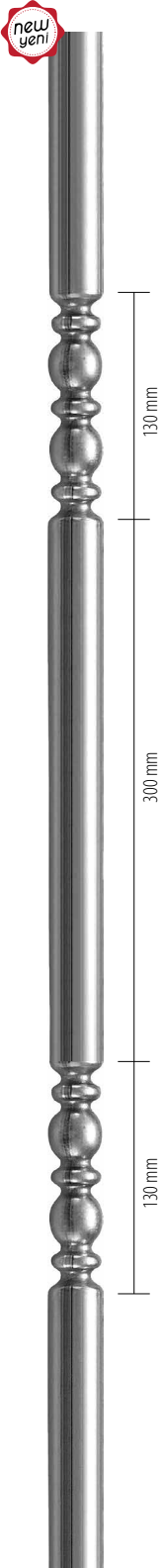
2029-A 1.2 mm Ø 32 mm 900 mm
