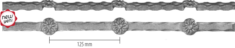
26106-B □ 12 mm 2000 mm
