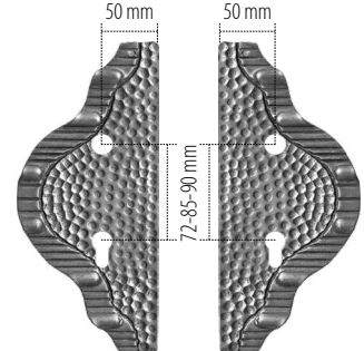
3959-A 120x290 mm 3 mm
