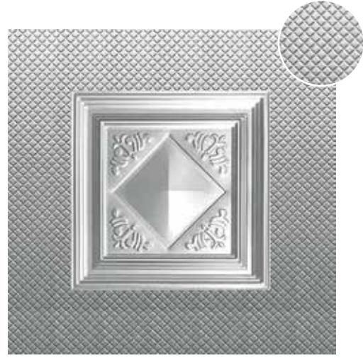
0491-A 1000 (520x520) x 1000 x 0.90 mm
