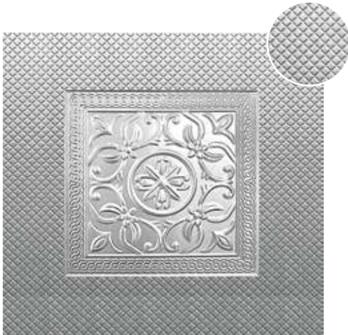
0497-A 1000 (520x520) x 1000 x 0.90 mm
