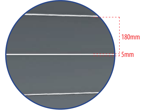
maksimum gizlilik-5mm boşluk maximum privacy-5mm gap
